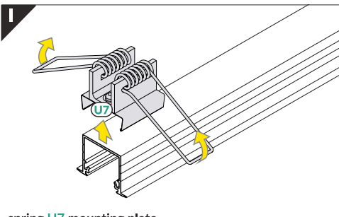
spring U7 mounting plate uchwyt U7 sprężyna
